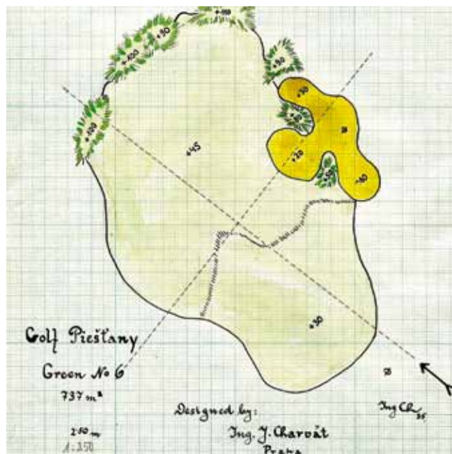
Charvátův návrh rekonstrukce greenu č. 6, 1935 (projekt z archivu GCP)
