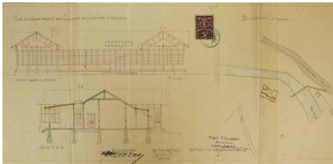
Plán nové klubovny v Gejzírparku/Stavební archiv Magistrátu Města Karlovy Vary.
